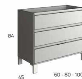
Detalle cajón
